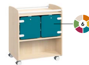
Meuble papier à dessins à portes L 784 x H 934 x P 565 mm - Portes équipées de serrures 2 étagères - 4 roues à frein - Livré monté (hors roues) Réf. G666
